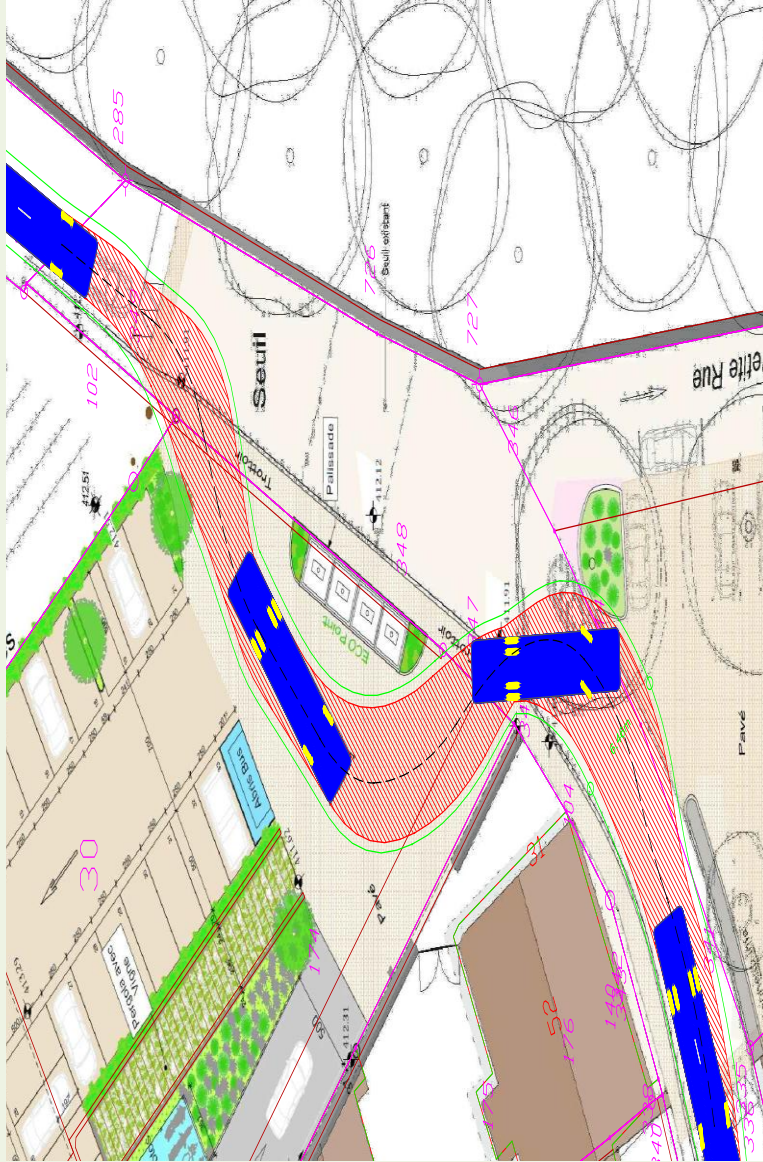
Place de la Croix, viabilité pour un bus de 12 m.
